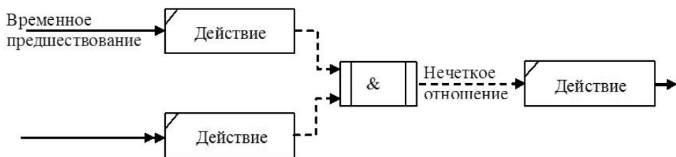
Рис. 3. Диаграмма IDEF3
